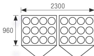
PBOX1824 Box 18 à 24 places L2300 x P960 x H2100mm Poids : 350 Kg
